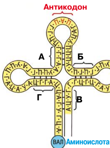
Вторичная структура тРНК (на примере валиновой)
