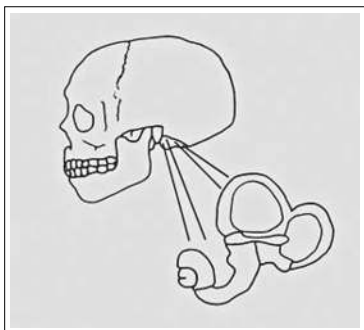
Полукружные каналы внутреннего уха человека
