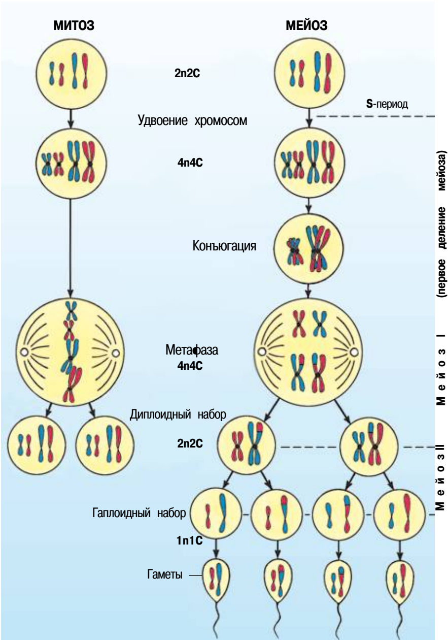
Поведение хромосом при митозе и мейозе. Гомологичные хромосомы на рисунке одинакового размера, отцовские и материнские хромосомы показаны различными цветами
