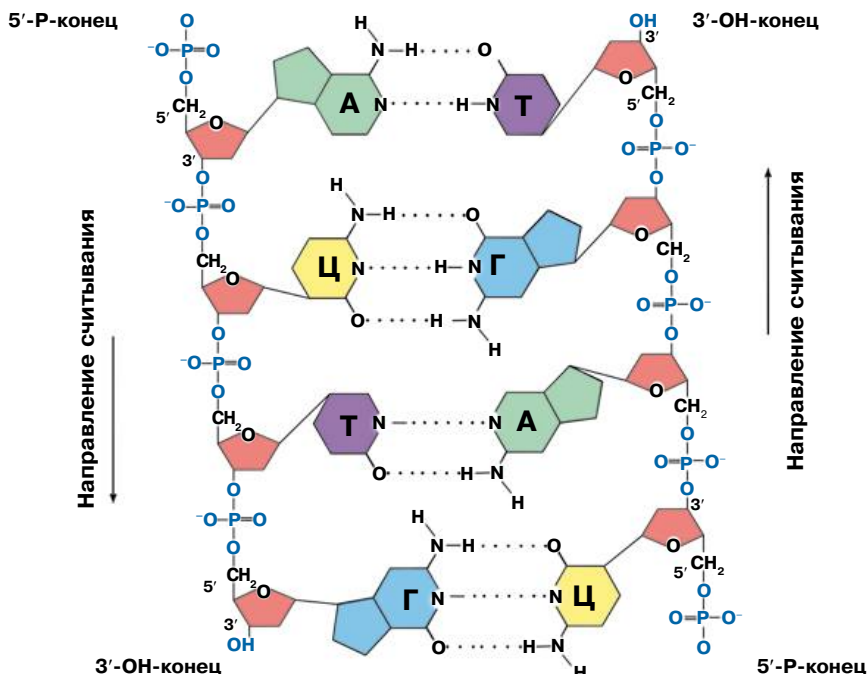
Участок двойной спирали молекулы ДНК
