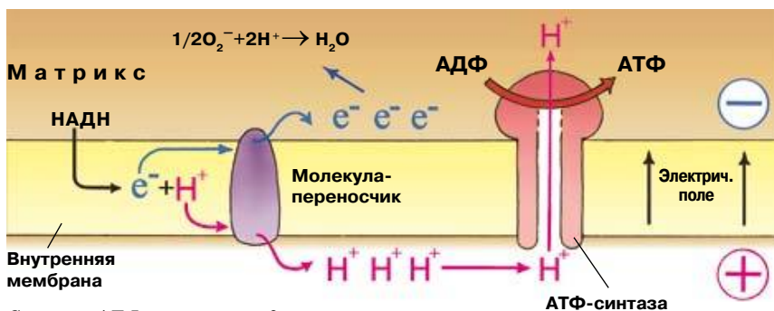
Синтез АТФ в митохондрии
