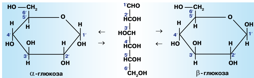
Глюкоза. Линейная форма и два циклических изомера
