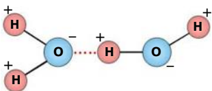
Образование водородной связи между молекулами воды
