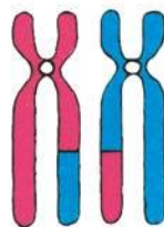
кроссинговер — перекрест хроматид в мейозе
