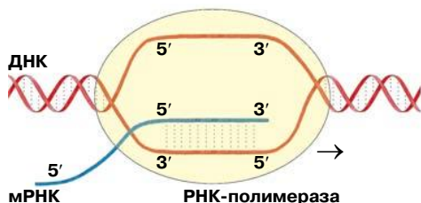
Схема транскрипции (транскрибируется нижняя нить ДНК слева направо)
