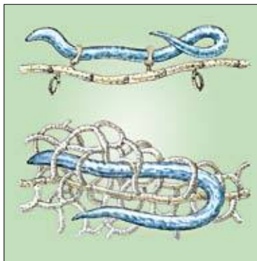
Хищничество у грибов
