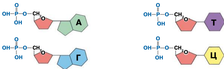
Четыре нуклеотида, входящие в состав молекулы ДНК
