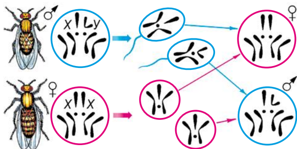
Схема расщепления по признаку пола у дрозофилы
