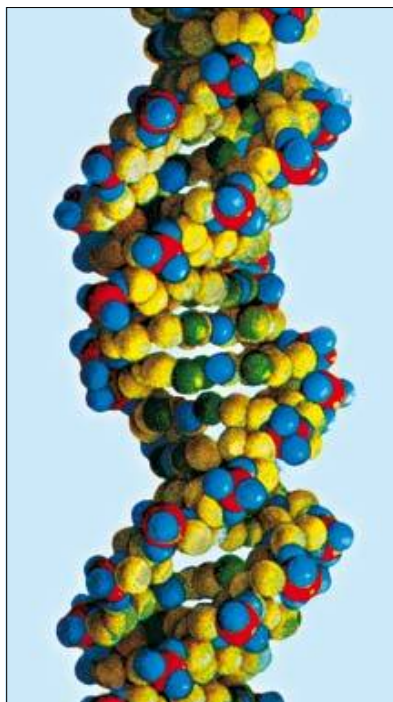
Двойная спираль ДНК
